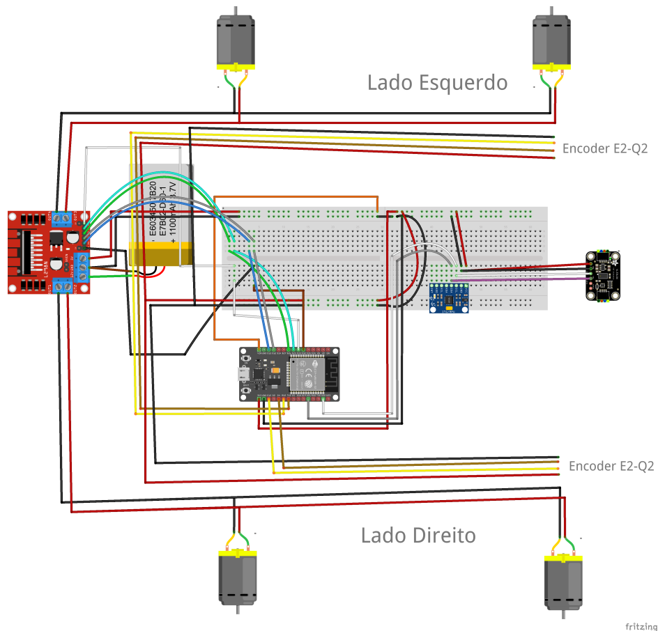
Figura 8 – Modelo do robô representado em placa de prototipação. Modelo desenvolvido com auxílio da ferramenta Fritzing.org .
